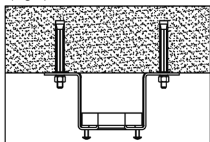
1-SOPORTE MONTAJE
